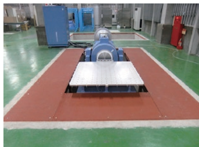
▲新規導入した大型振動試験機 対応可能な貨物のサイズは、重量約1,000kg、パレットサイズ1,500mm × 1,500mm × 高さ 約2m まで
